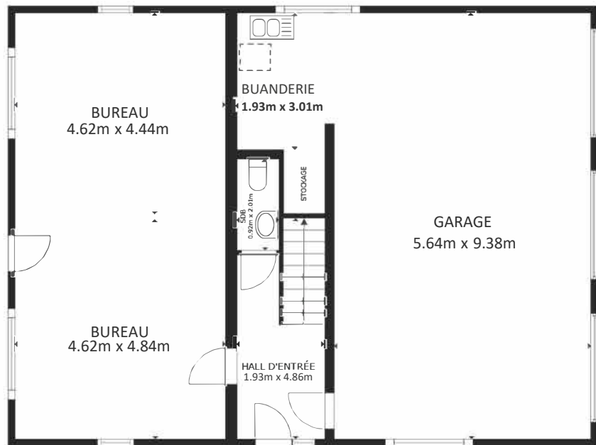
REZ-DE-CHAUSSEE
