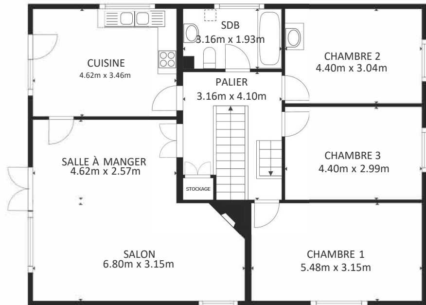
1ER ETAGE
